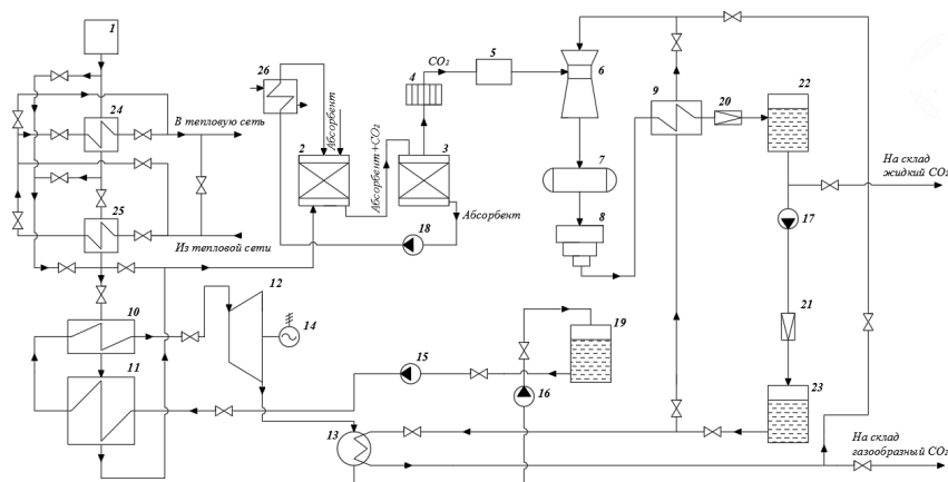
Рис. 1. Схема детандерной установки с производством жидкой и газообразной углекислоты:
