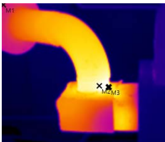
Рисунок 1 – Термограмма дымохода на выходе из котла КС-ТГ
