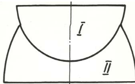
Рис. 6. Зоны деформации при осаживании цилиндрических образцов
