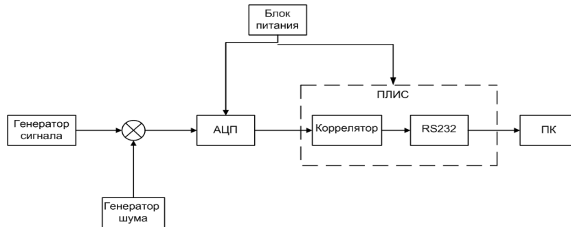
Рис. 4. Схема эксперимента
