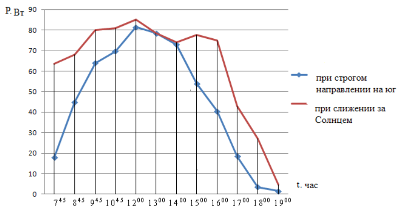
Рис. 3. График зависимости изменения вырабатываемой мощности по времени
