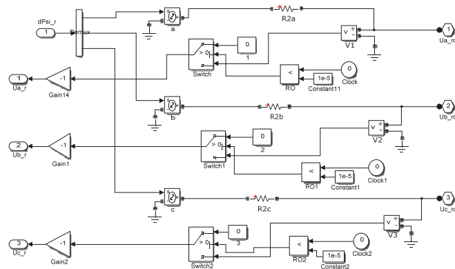
Рис. 2. Параметры блока связи силовых клемм роторной цепи с сигналами имитационной модели асинхронной машины в Matlab Simulink
