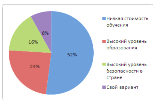
Рис. 4. Причины поступления
