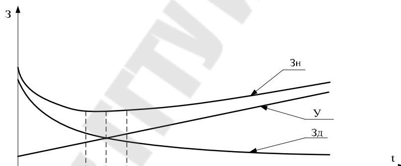
Рис. 2. Зависимость ежегодной стоимости ущерба ( Y ) от недоотпуска электроэнергии и дополнительных затрат ( Z_d ) на повышение надежности от средней ежегодной длительности перерывов электроснабжения
